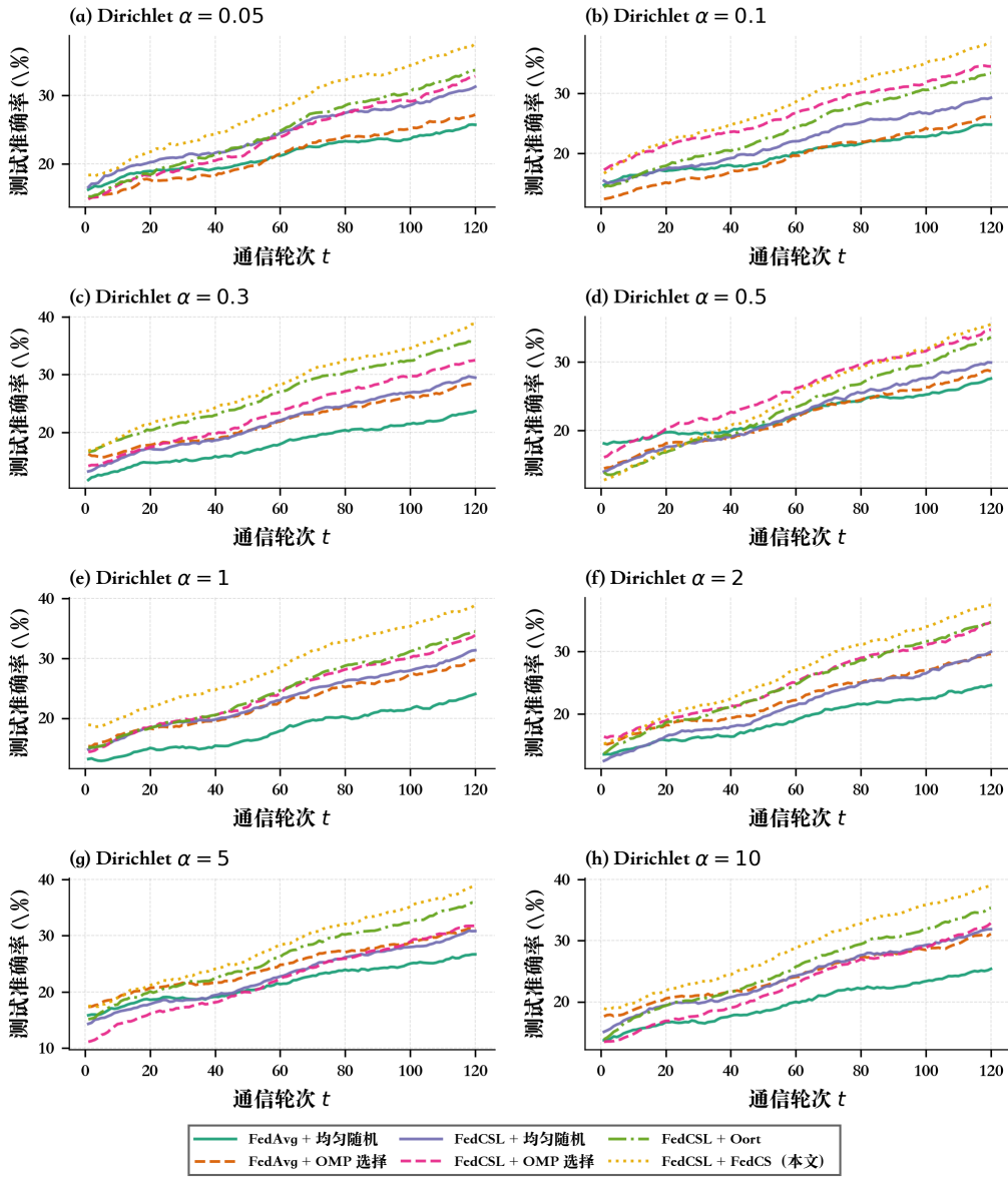
Figure 4: 不同 Dirichlet 参数 \alpha 下各尺度选择策略的测试准确率随 round 变化曲线 (4×2 子图: 自上而下、自左而右依次对应从强异构到弱异构的 \alpha 取值)。
